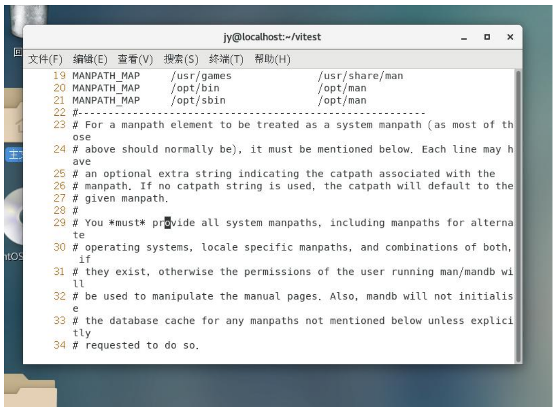
图 11 按 29G 到 29 行, 再按 15l 到第 15 个字符, 再按 i 进入插入模式删除字符
